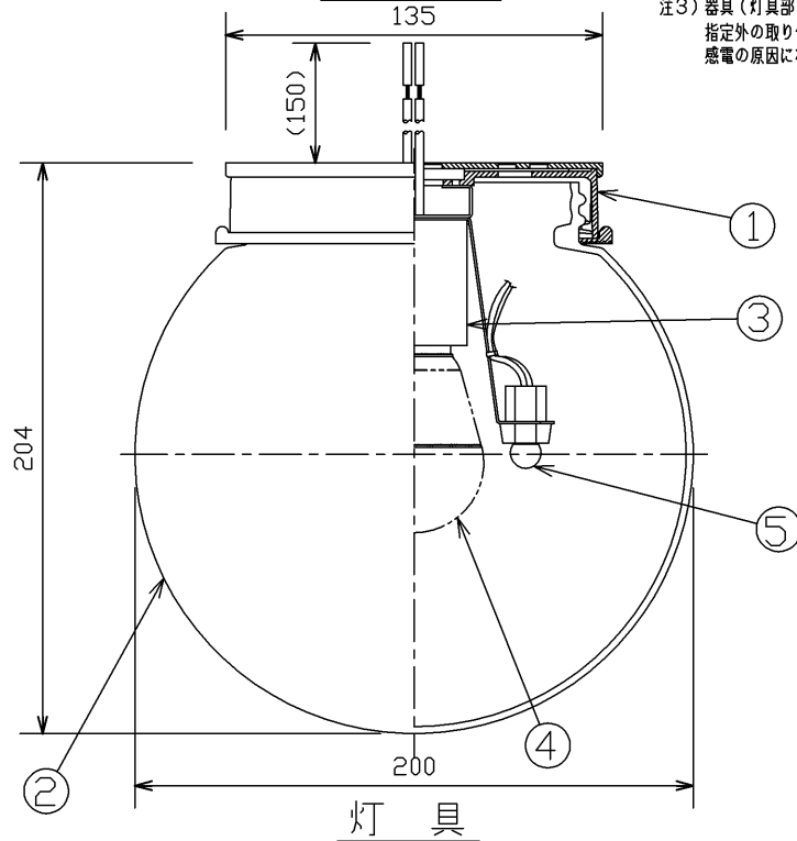
背面取付け図
