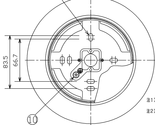
背面取付け図
