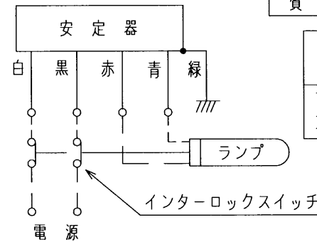
結線図
