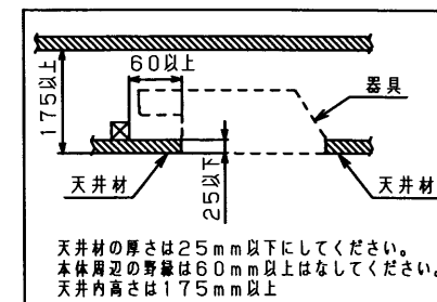
天井施工上の注意
