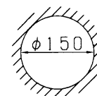
埋込穴寸法 天井取付厚さ: 5~25mm
