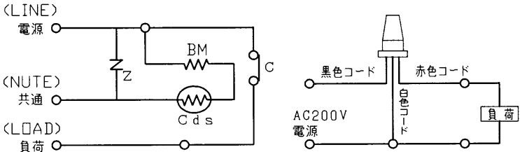
内部結線図
