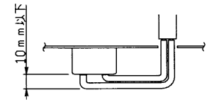
VVFケーブルの端子台接続寸法 反射板との当たりを防ぐため10mm以下になるように配線してください。
