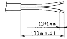
VVFケーブルの曲みきり寸法
