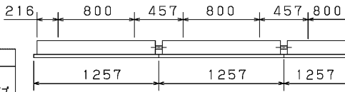
連結使用例
