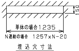
埋込穴寸法
