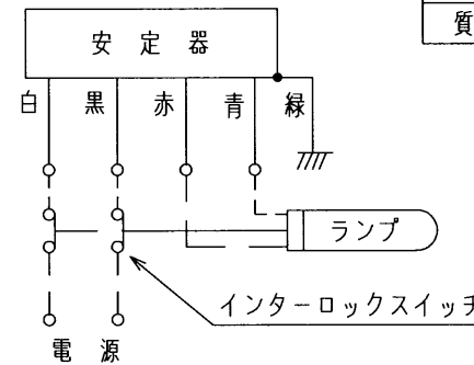
結線図
