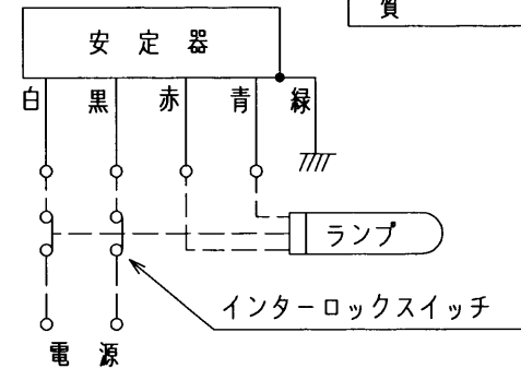
結線図
