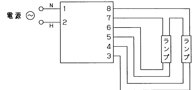
結線図
