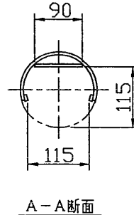
安定器収納部 詳細図 (蓋は除く)
