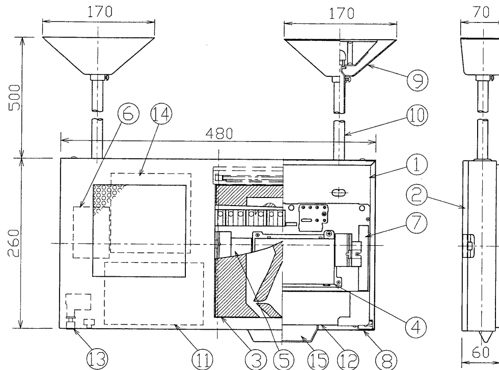
取付寸法図
