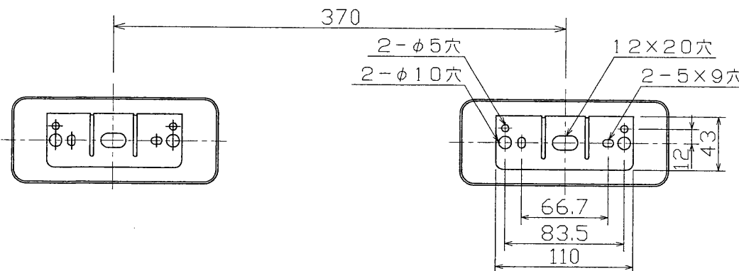
取付寸法図
