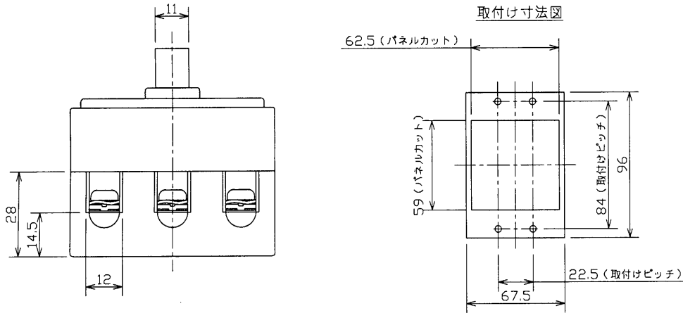
取付け寸法図
