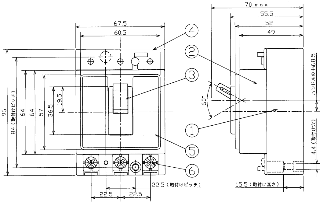
取付け寸法図
