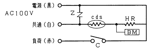
内部結線図
