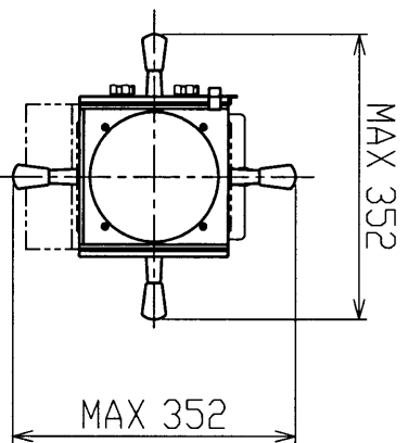
カッター板 全開状態寸法
