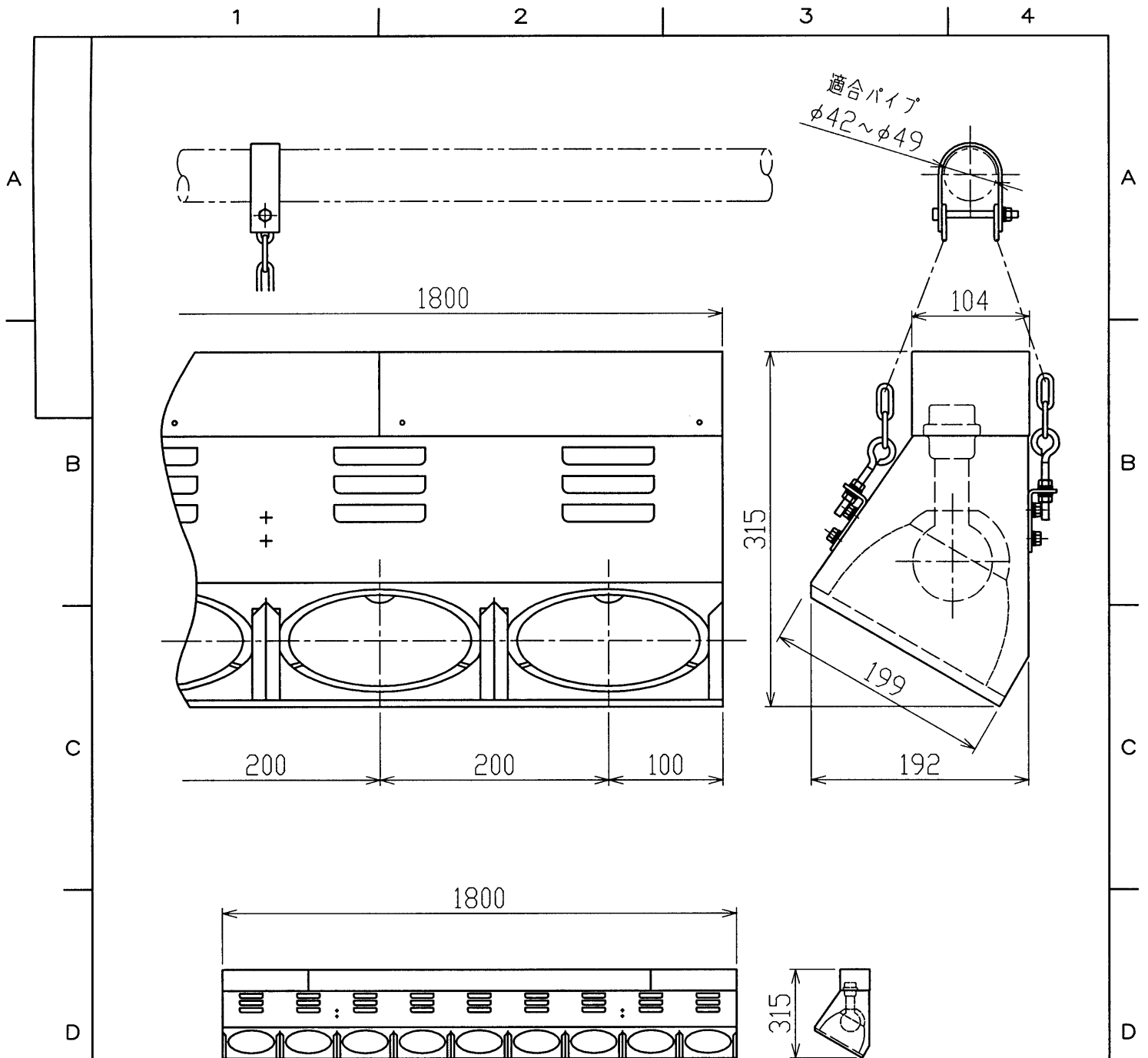
全体図 尺度=1/20
