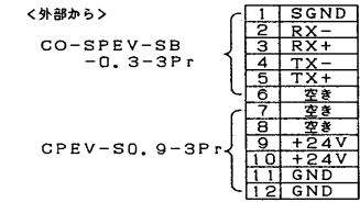
端子台 (TB)
