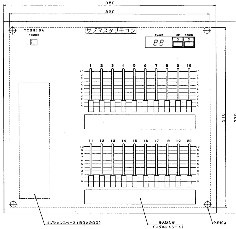
外觀図
