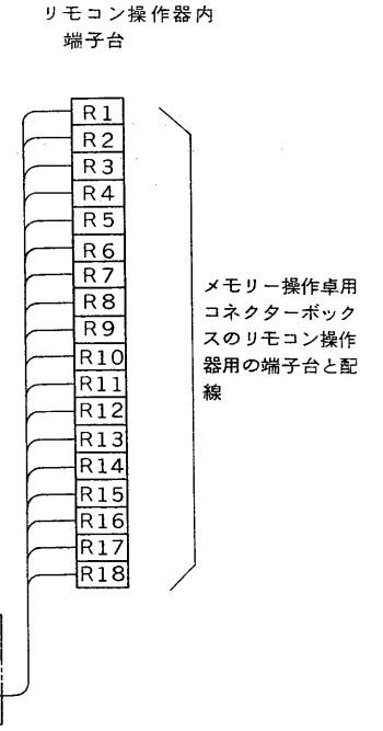
結線図
