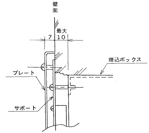
取付詳細図 (1/1)
