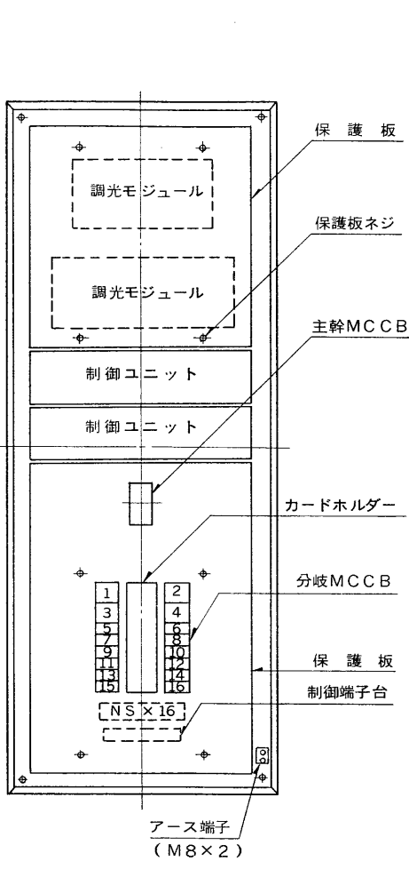
機器配置図
