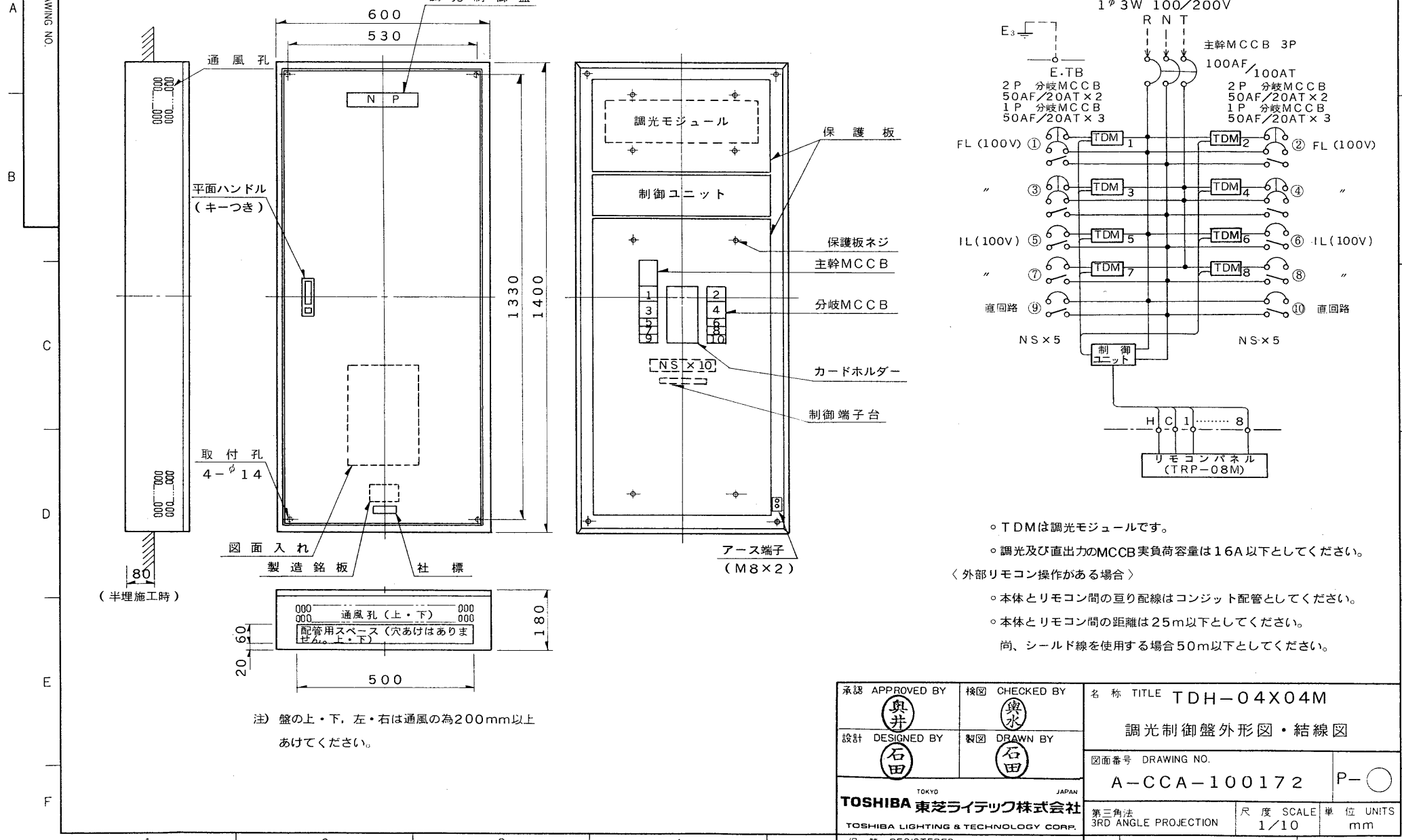
結線図
