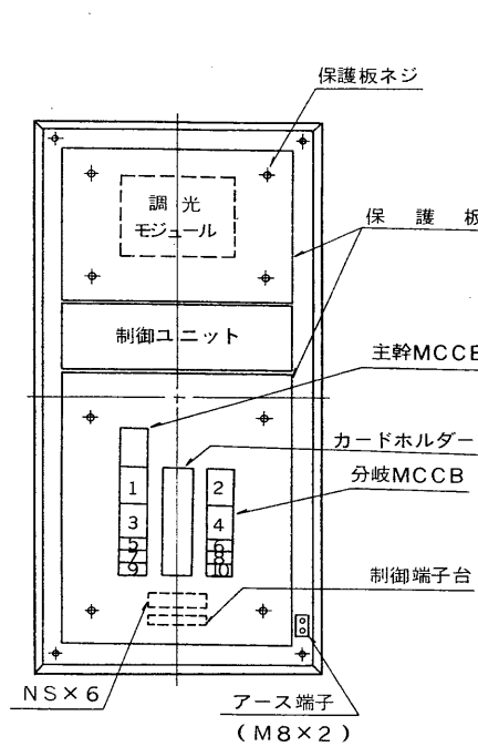
機器配置図
