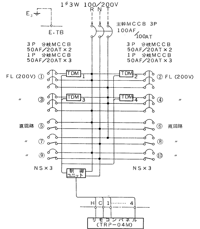
結線図
