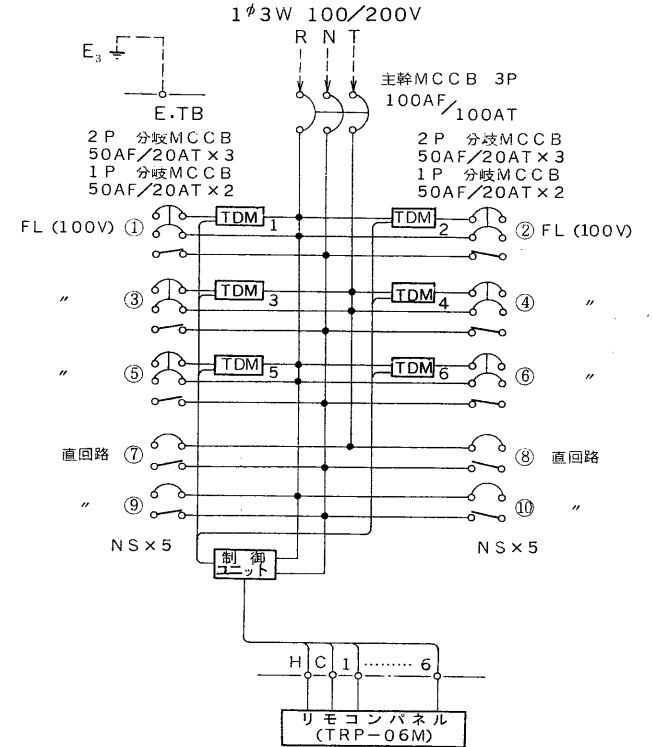
結線図
