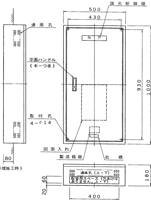
外形図
