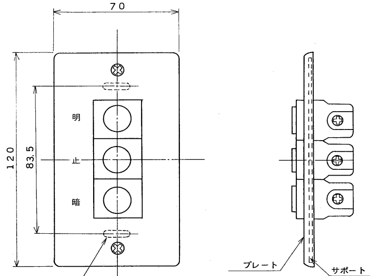
参考組立図
