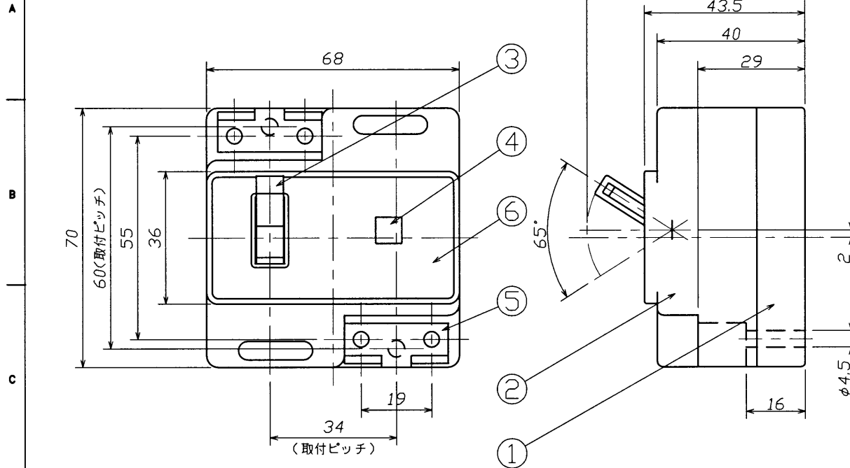
取付寸法
