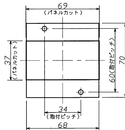
取付寸法
