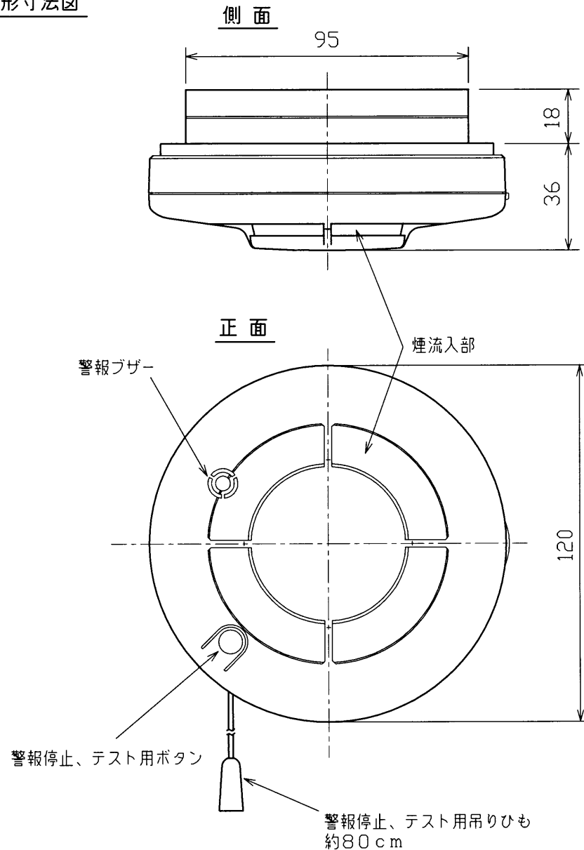
外形寸法図
