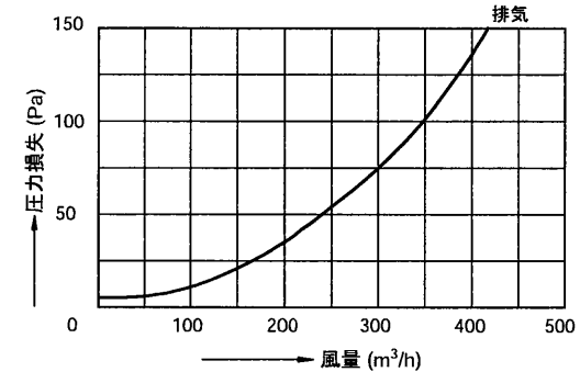
●圧力損失曲線
