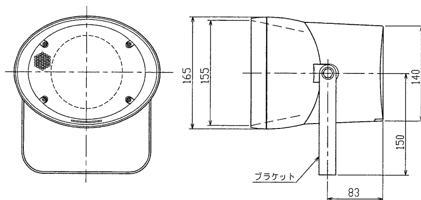
ブラケット取付寸法図
