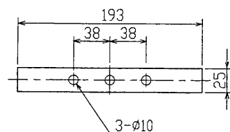
ブラケット取付寸法図
