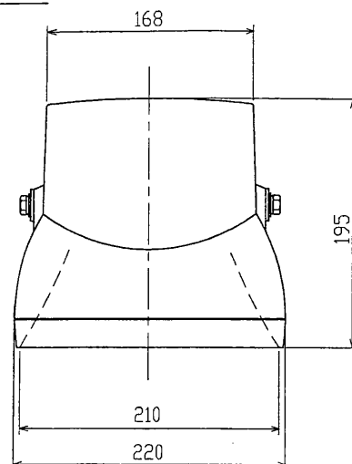
外観寸法図
