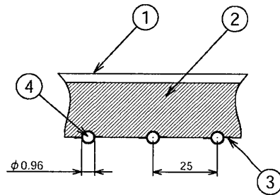
断面詳細図
