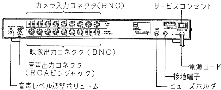
(背面図)
