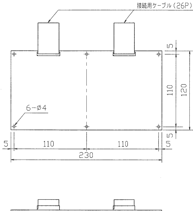
外觀寸法図
