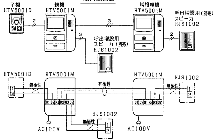
最大接続図
