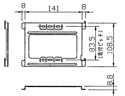
取付金具 (t1.6)
