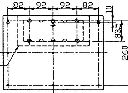
スイッチボックス取付穴寸法
