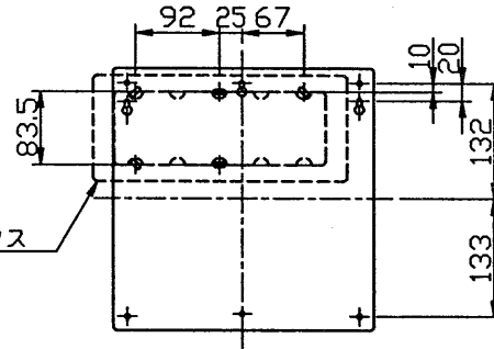
スイッチボックス取付穴寸法
