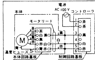
結線図
