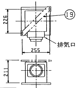
■吊下金具(別売部品) 取付位置
