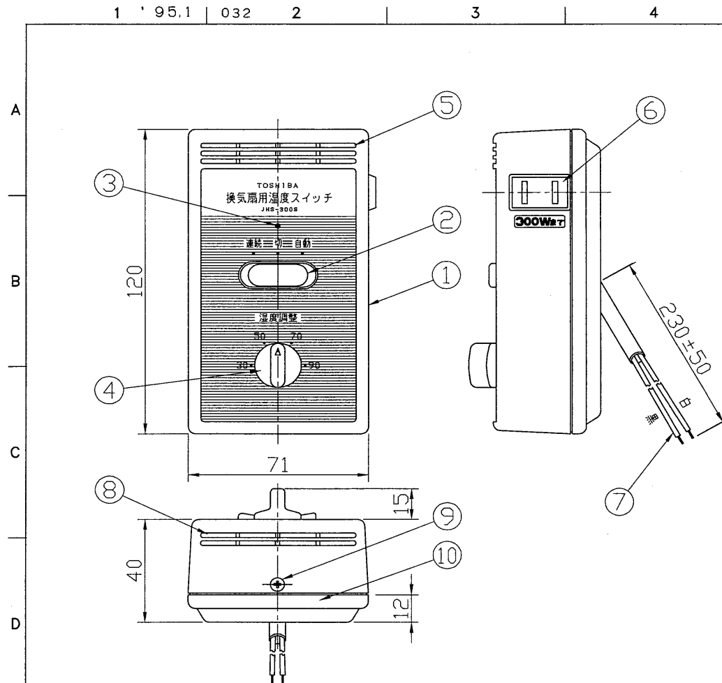
構成図
