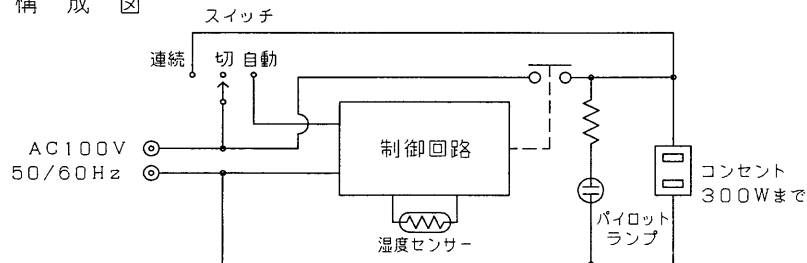
構成図
