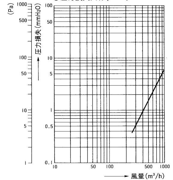
●圧力損失曲線(φ300)
