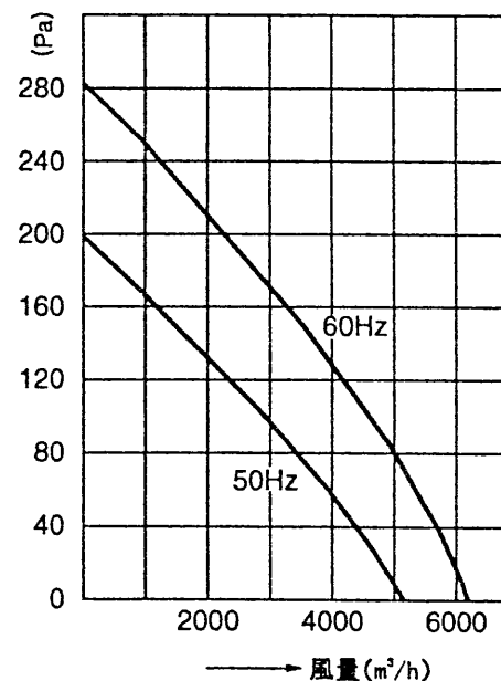
■ 静圧 - 風量特性
