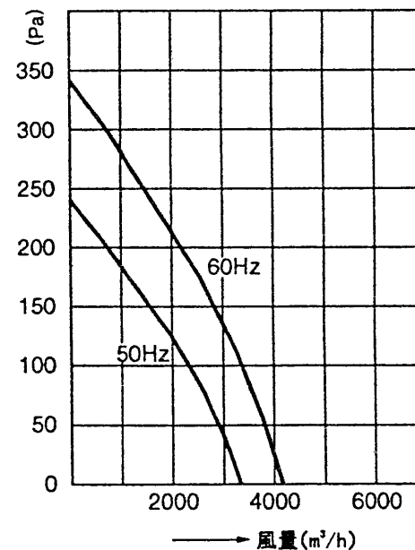
■ 静圧－風量特性
