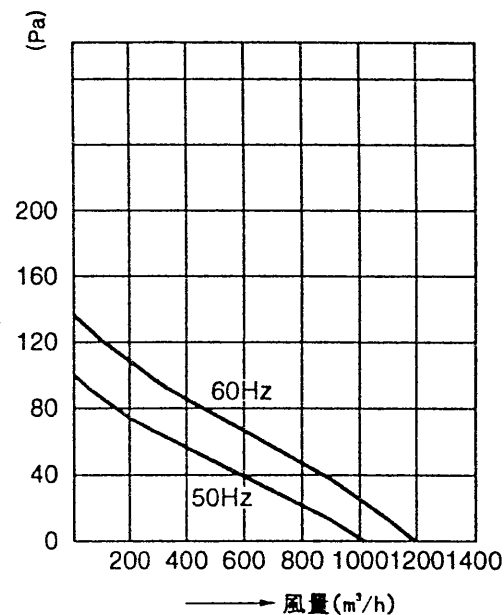
■ 静圧 - 風量特性
