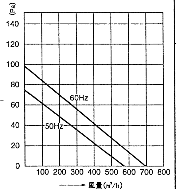
■ 静圧－風量特性
