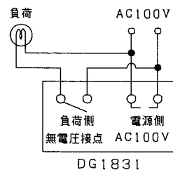
配線例（100V照明器具）
