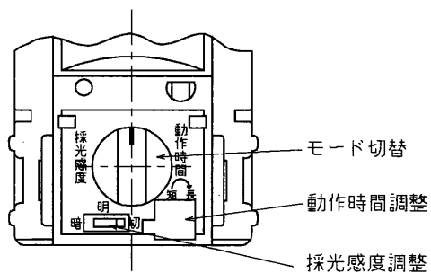
化粧カバーを外した状態
