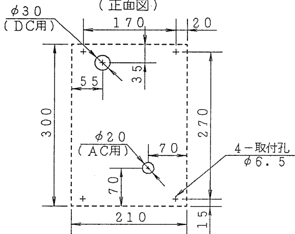
通線孔位置及び取付孔位置 (正面図)
