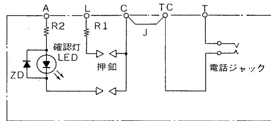
回路図
