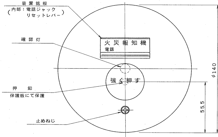
取付寸法図
