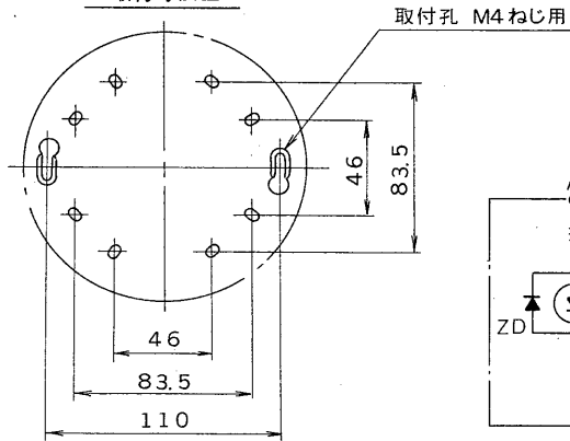
取付寸法図
