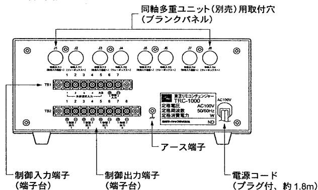
〔背面図〕
