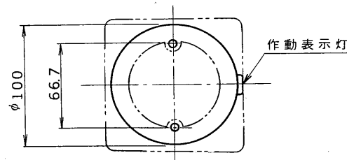
取付寸法図
