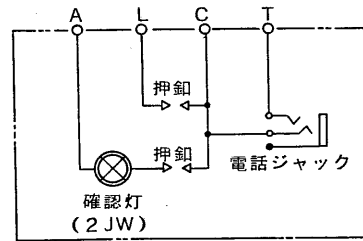
回路図
