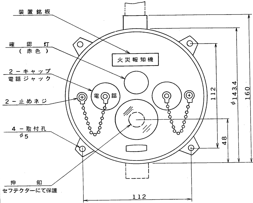
外觀寸法図
