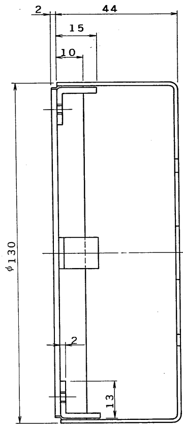
A - A 断面図
