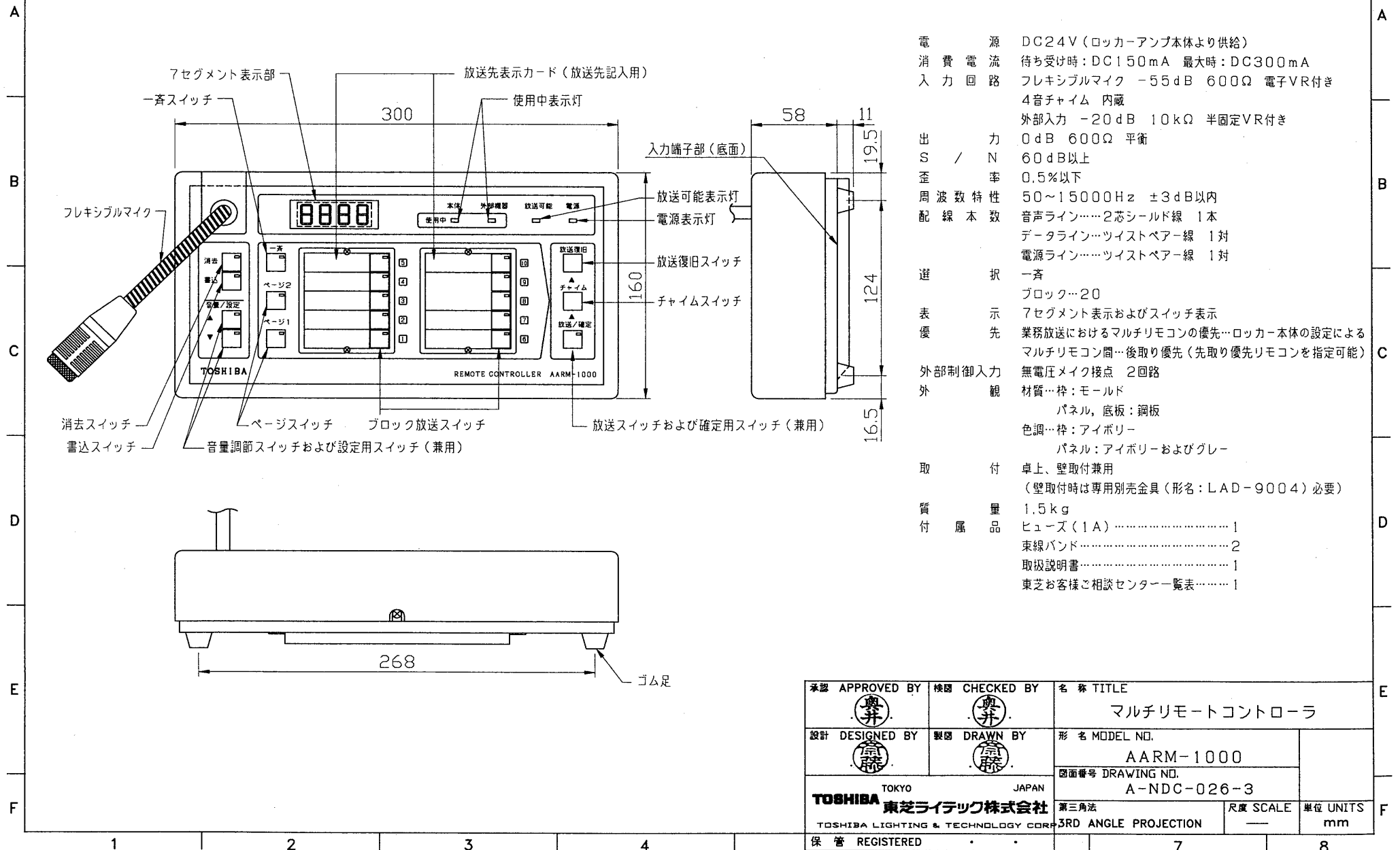
外観寸法図
